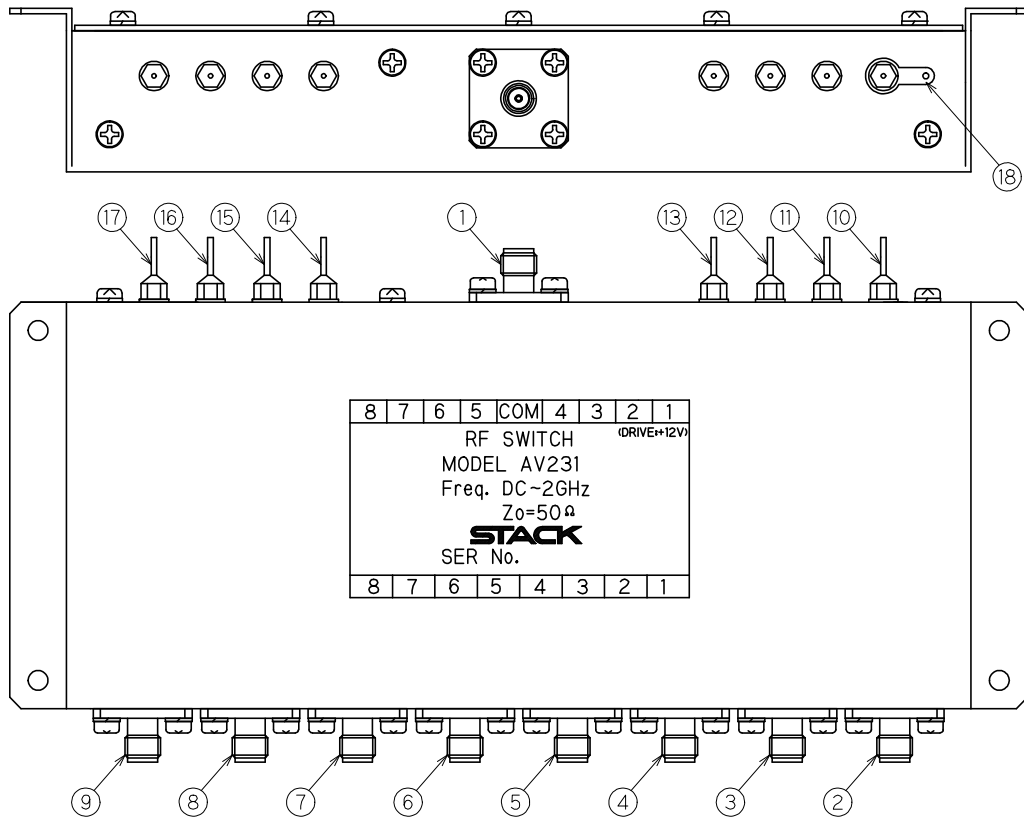
図2 本体機能図
