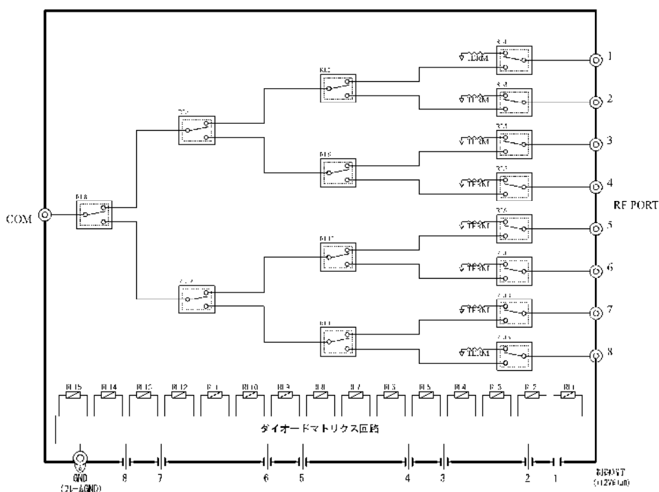
図 1 回路図
