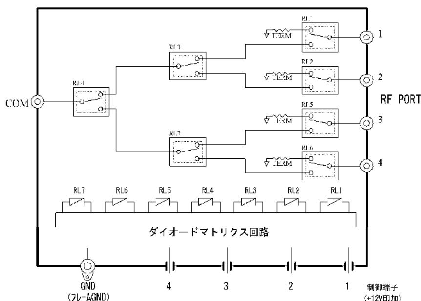
図 1 回路図
