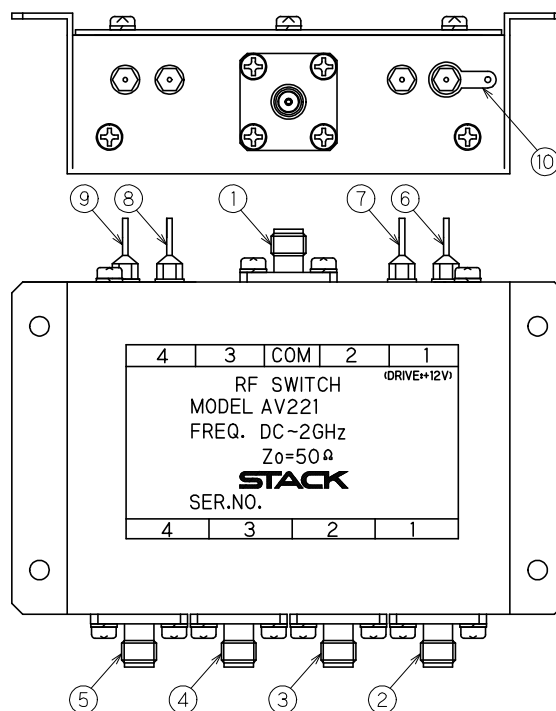
図 2 本体機能図
