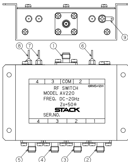
図 2 本体機能図
