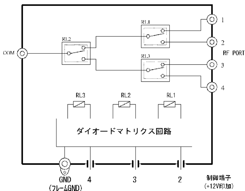
図 1 回路図
