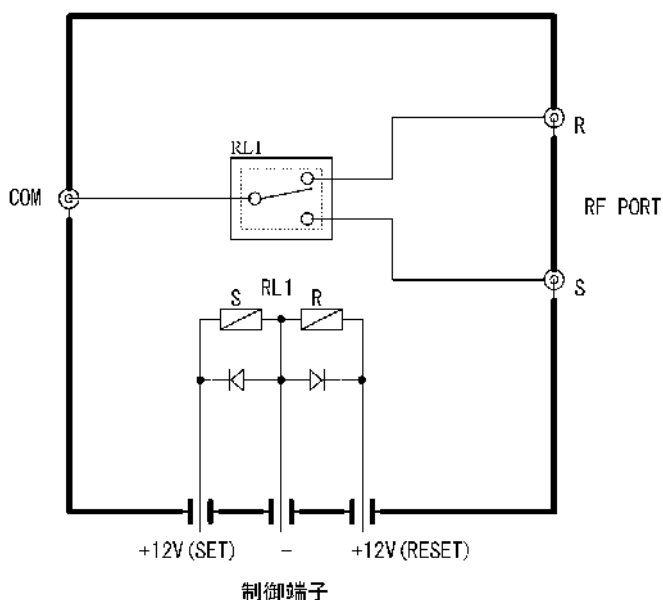
図 1 回路図
