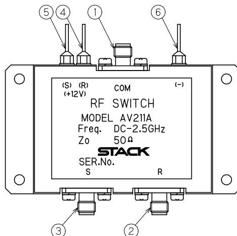
図 2 本体機能図
