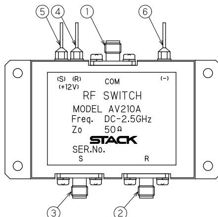
図 2 本体機能図
