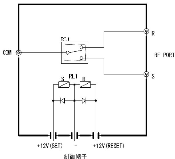
図 1 回路図
