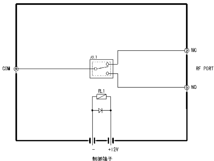
図 1 回路図
